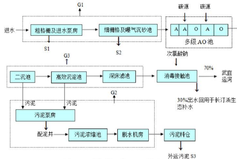
图 4-1 滨湖污水处理厂工艺流程图
